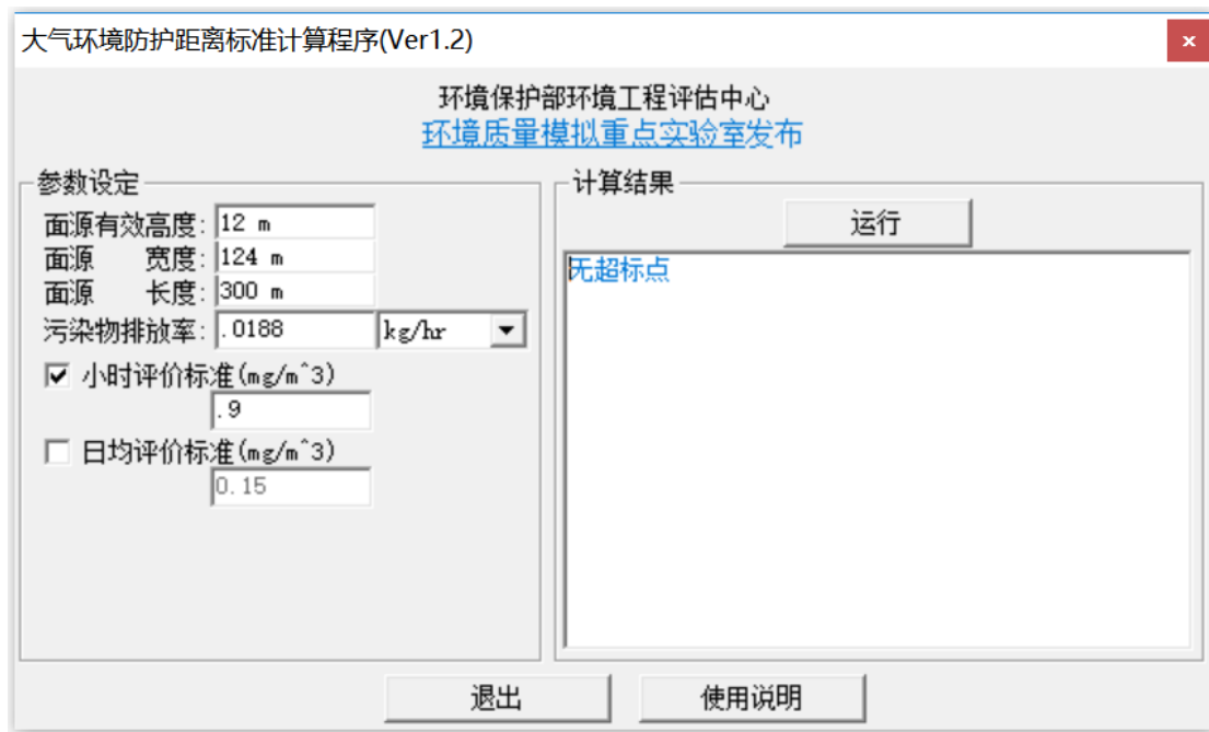
图 5-2-1 采场采剥无组织粉尘大气防护距离截图
