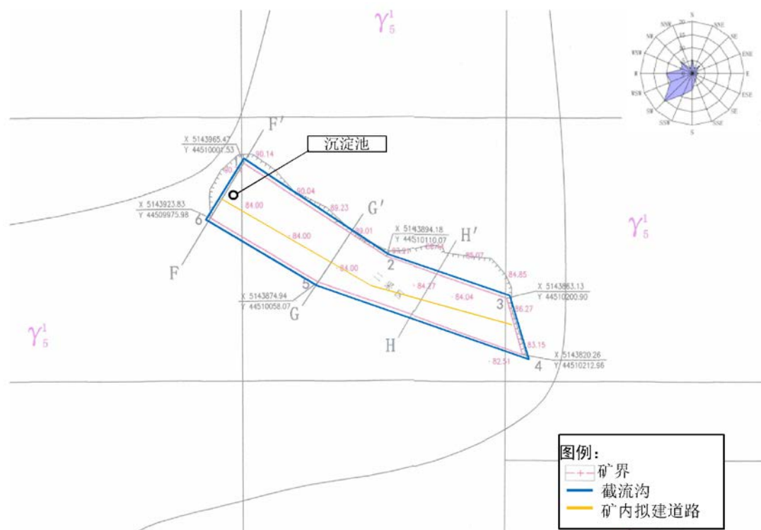
图 3-1-1 项目二采区平面布置图
