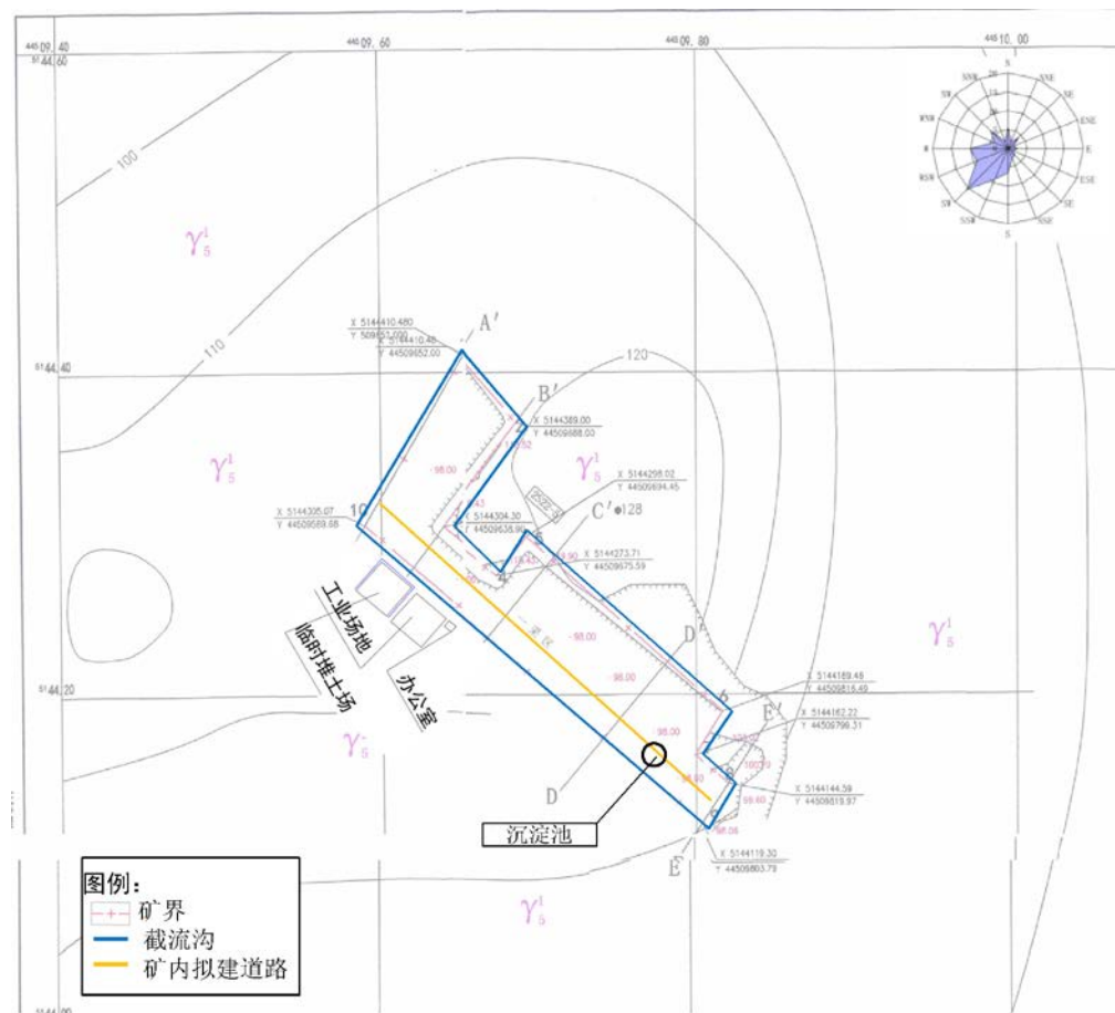
图 3-1-1 项目一采区平面布置图
